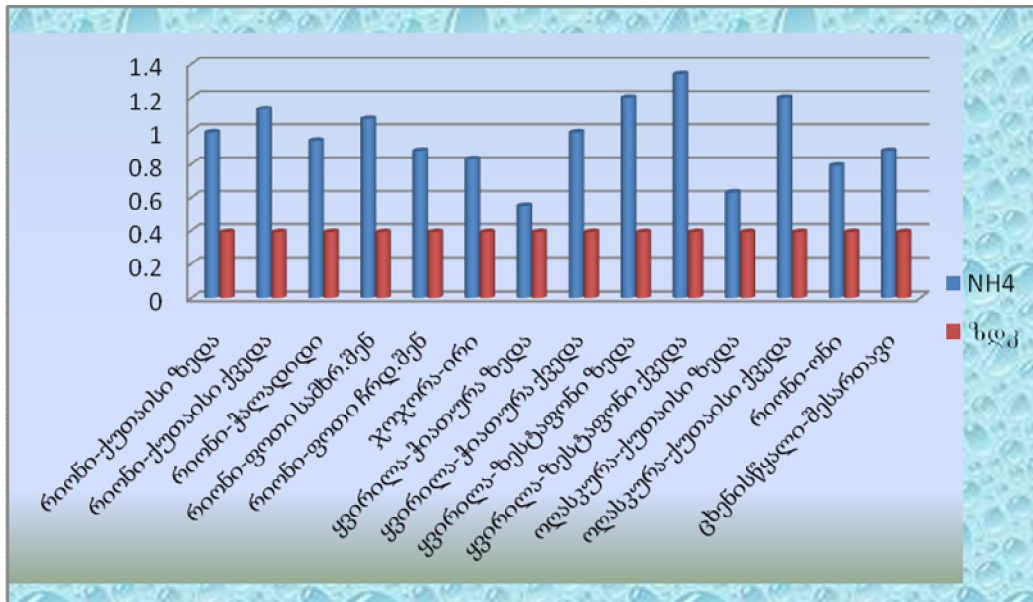
ნახ.10 მდ.რონი და მისი შენაკადები - NH 4 , ივლისი, 2013
