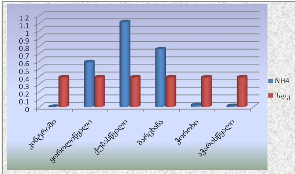
ნახ.11 აჭარა - NH 4 , ივლისი, 2013
