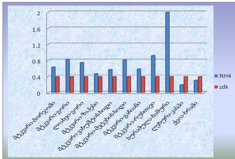
ნახ.13 მდ.მტკვარი და მისი შენაკადები - NH4, ივლისი, 2013
