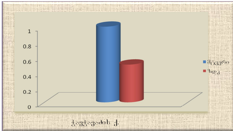
ნახ.3 მტვერის ერთჯერადი მაქსიმალური კონცენტრაცია, მგ/მ³
