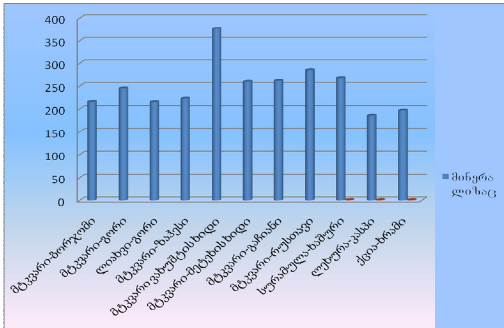
ნახ.12 მდ.მტკვარი და მისი შენაკადები - მინერალიზაცია, ივლისი, 2013
