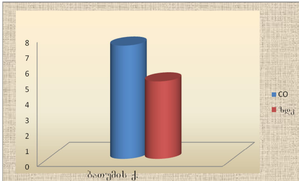
ნახ. 9 ნახშირყანვის ერთჯერადი მაქსიმალური კონცენტრაცია, მგ/მ 3
