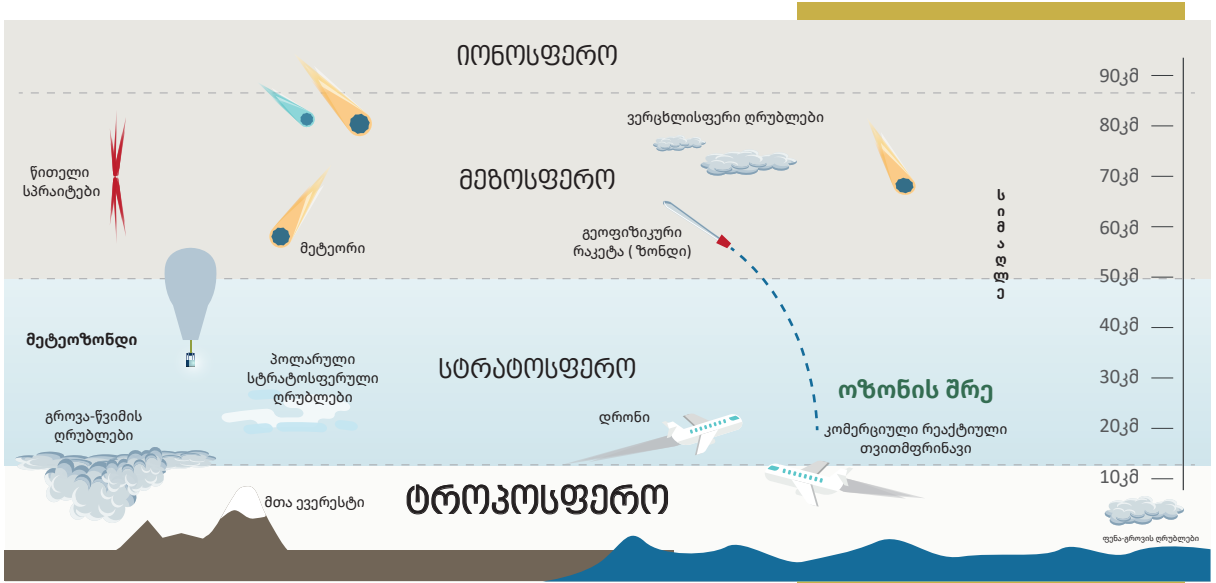
სურათი 1: ტროპოსფერო
